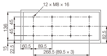
①SGLFW2-1DA380AS
